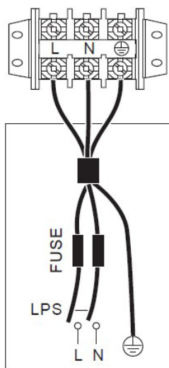
Připojení jednofázových verzí
