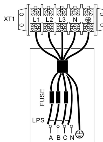
třífázový přívod
